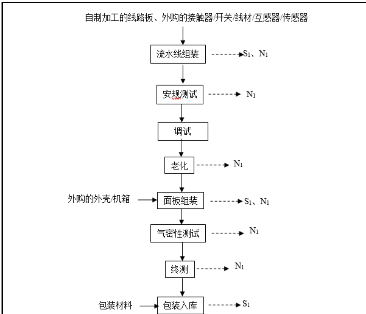
图 2-3 整机组装流程（位于一楼）
