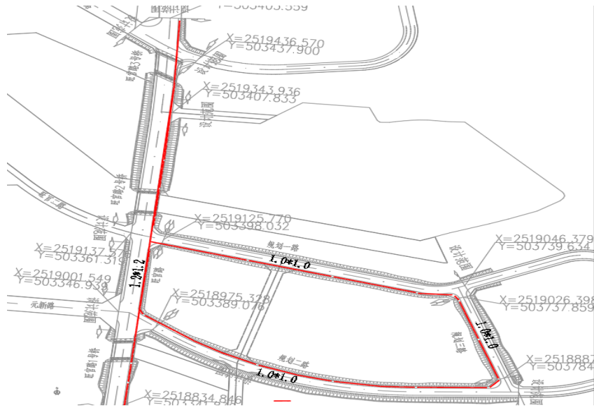
图 2-13 道路电力规划图
