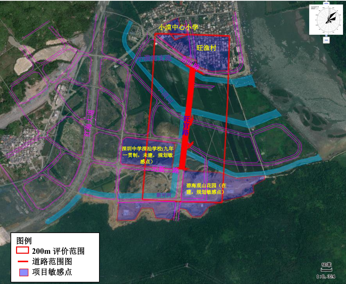
附图3 项目环境保护目标图
