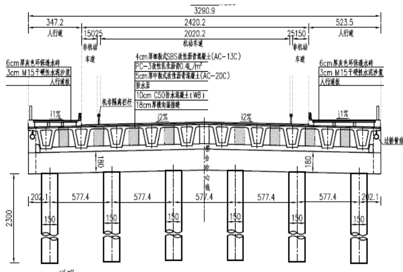
图 2-10 旺官路 3 号中桥横断面布置图
