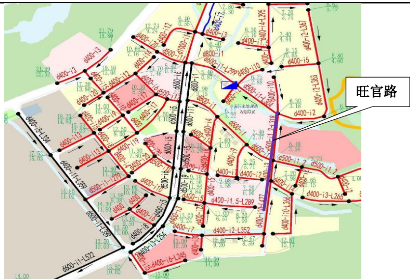
图 2-12 市政详规污水工程
