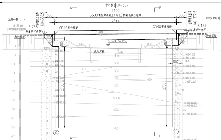
图 2-7 旺官路 2 号中桥桥梁桥型布置图
