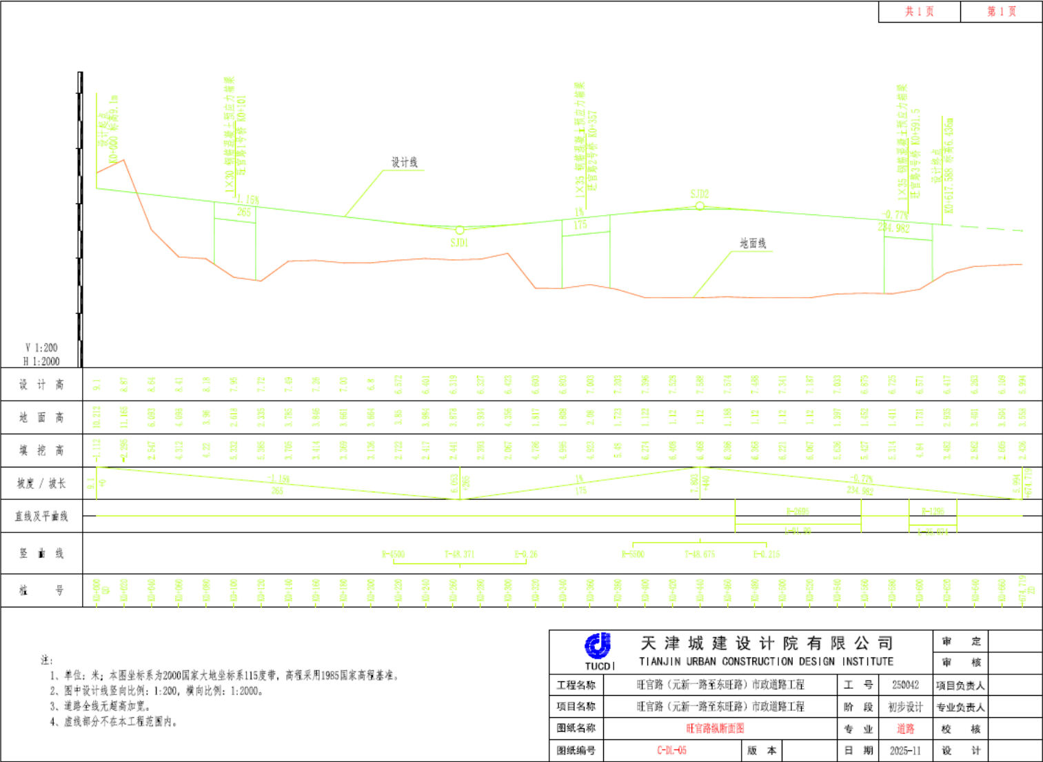
附图16 道路纵断面设计图
