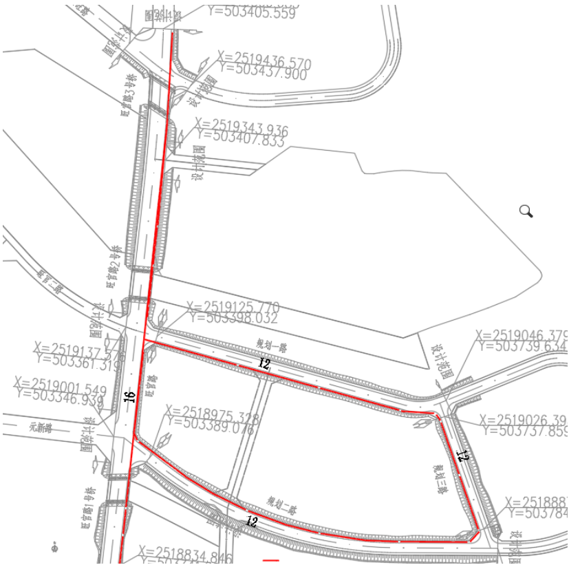
图 2-14 道路通信规划图
