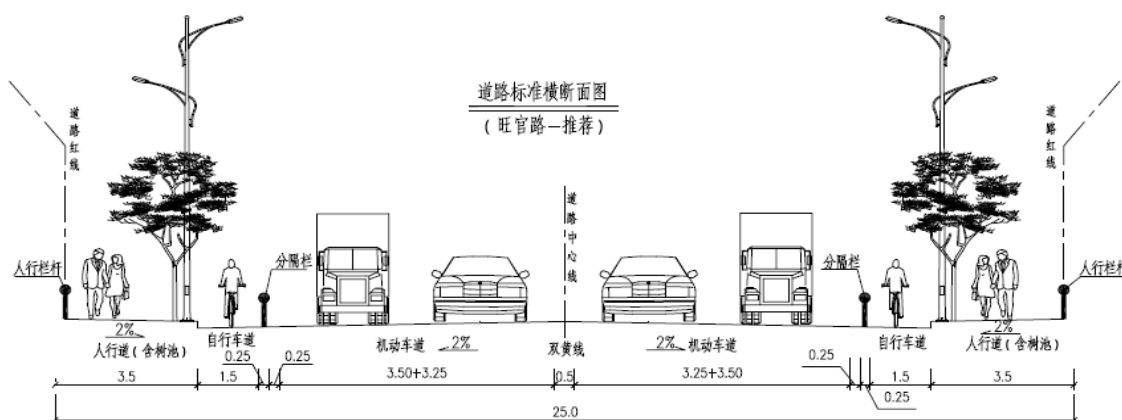
图 2-4 旺官路 25m 标准横断面图
