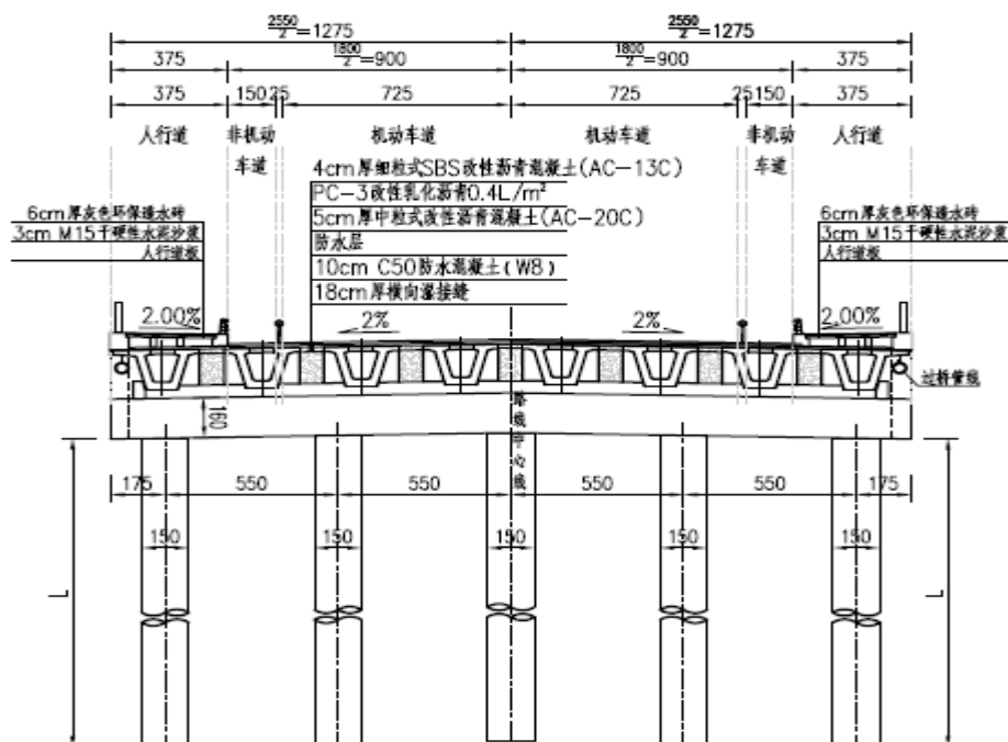
图 2-6 旺官路 1 号中桥横断面布置图
