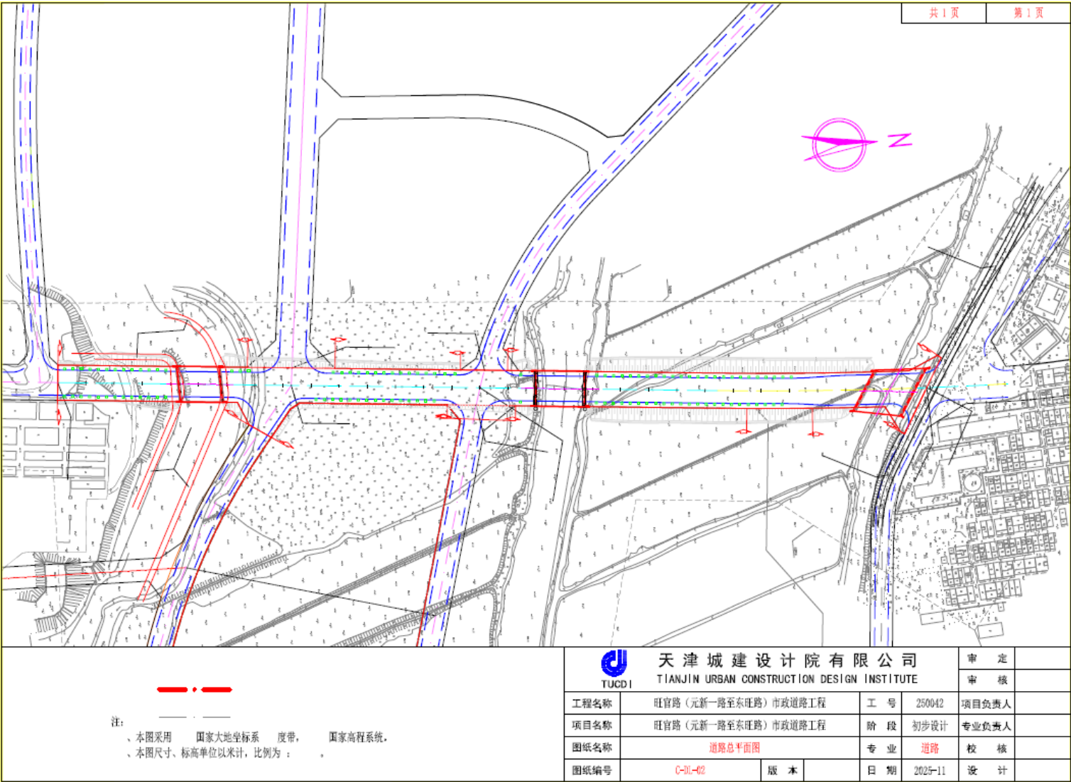
附图15 道路总体平面设计图
