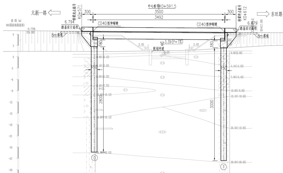
图 2-9 旺官路 3 号中桥桥梁桥型布置图
